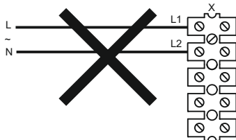
Anschlusschema 4
