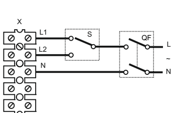
Anschlusschema 6
