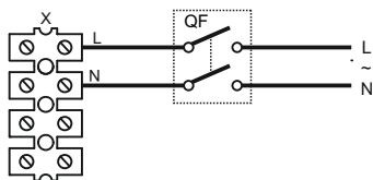
Anschlusschema 17
