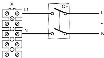
Anschlusschema 6
